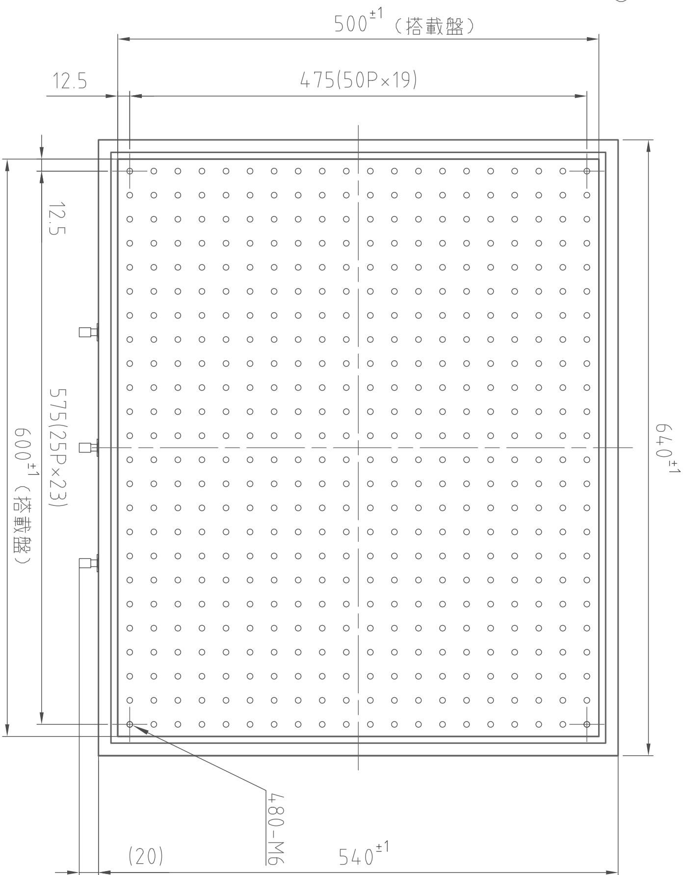
(平面図)
