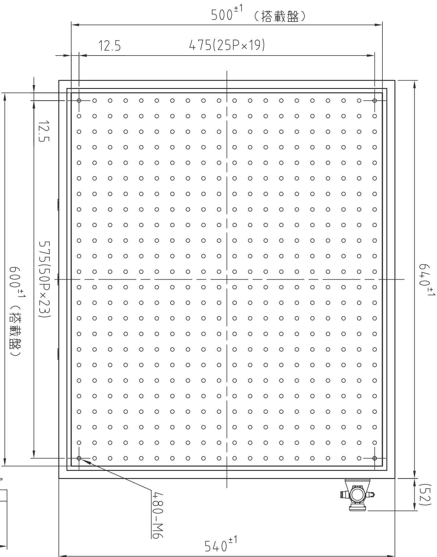
(平面図)
