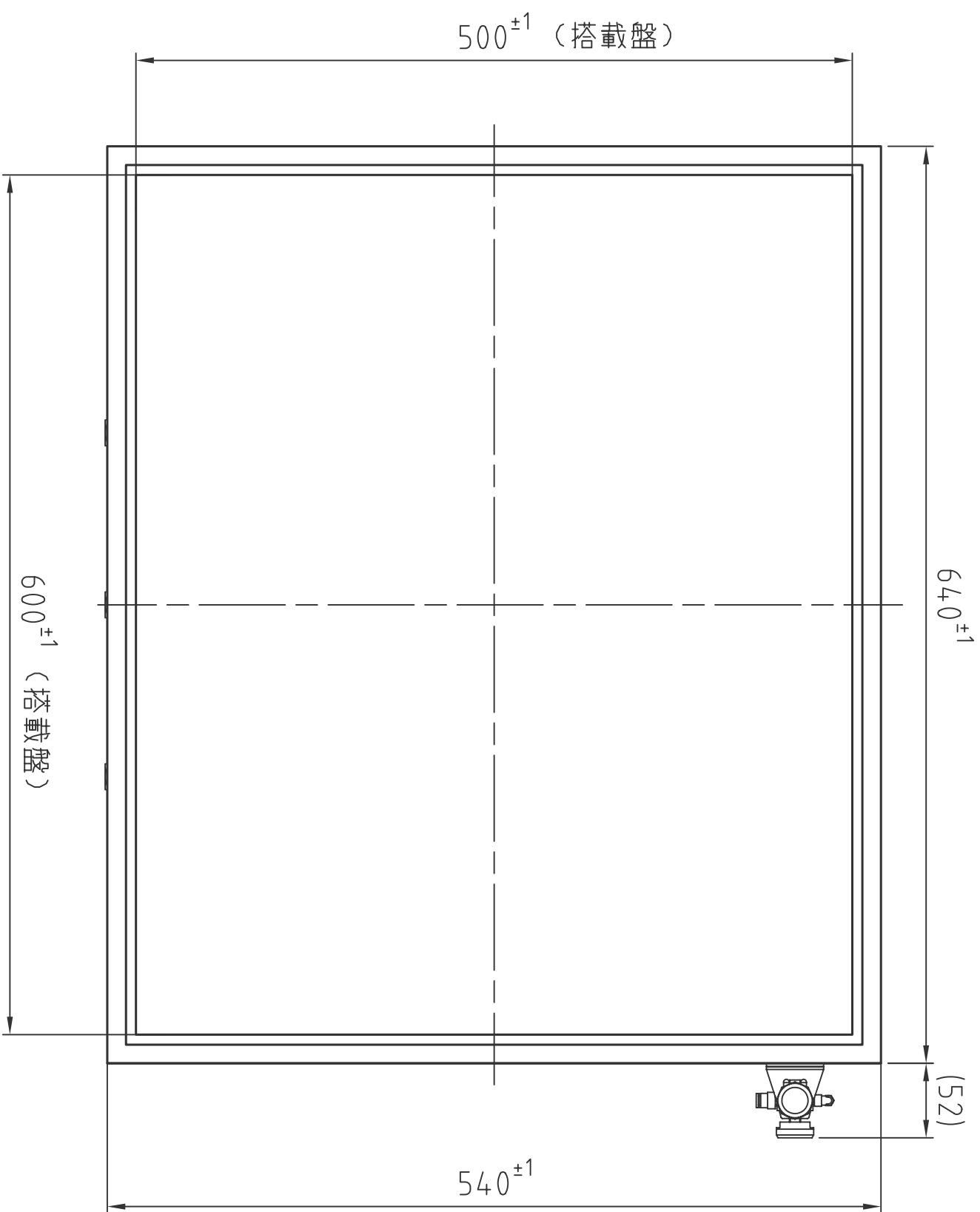
(平面図)
