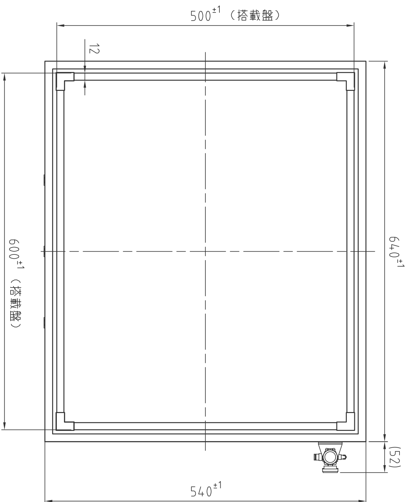
(平面図)
