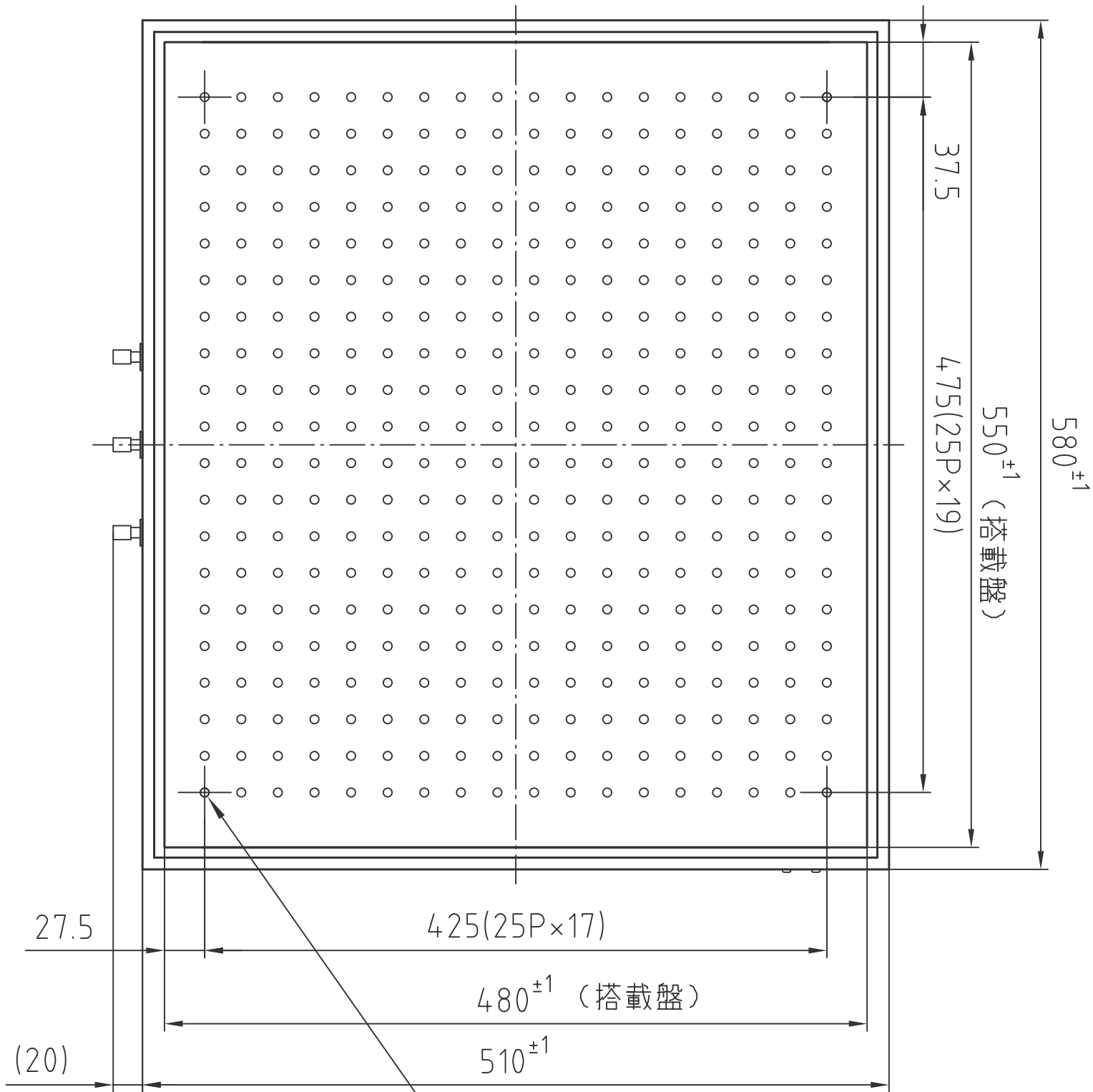
(平面図)
