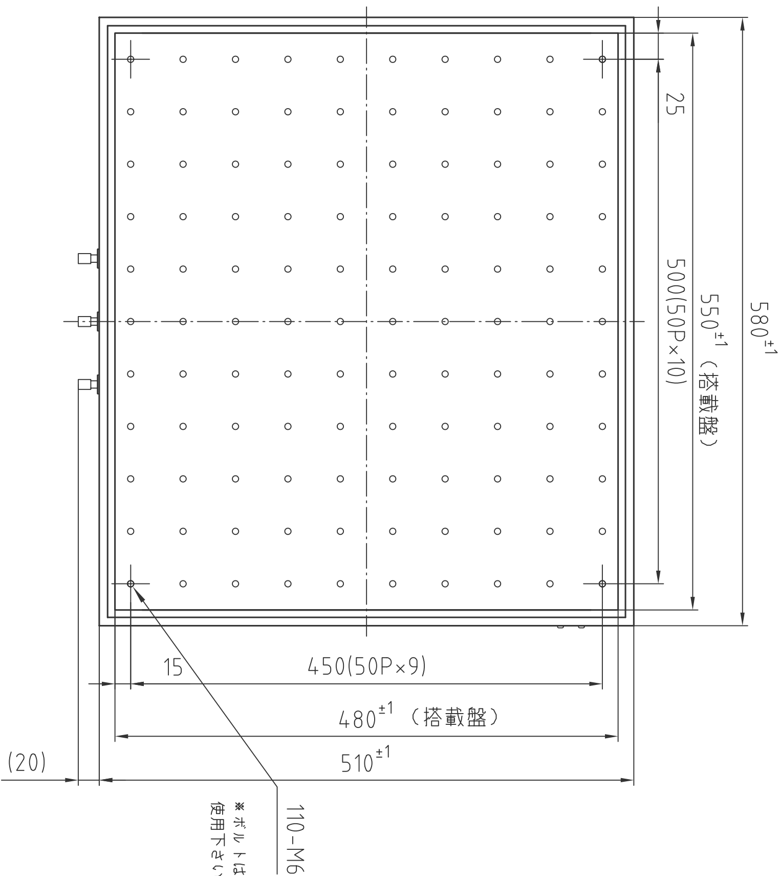
(平面図)
