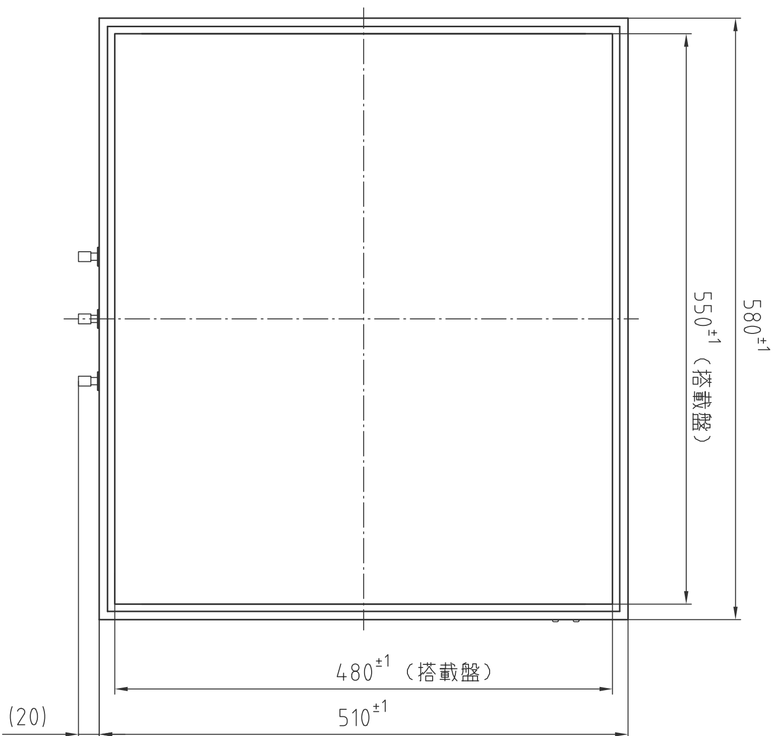
(平面図)
