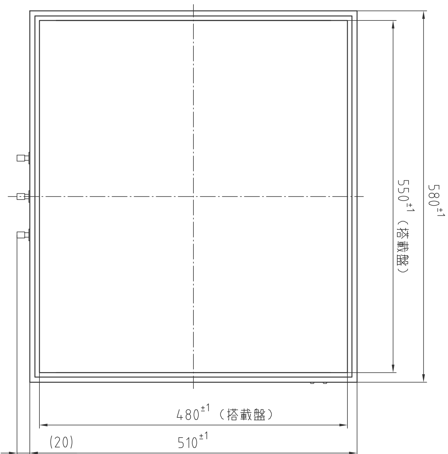
(平面図)
