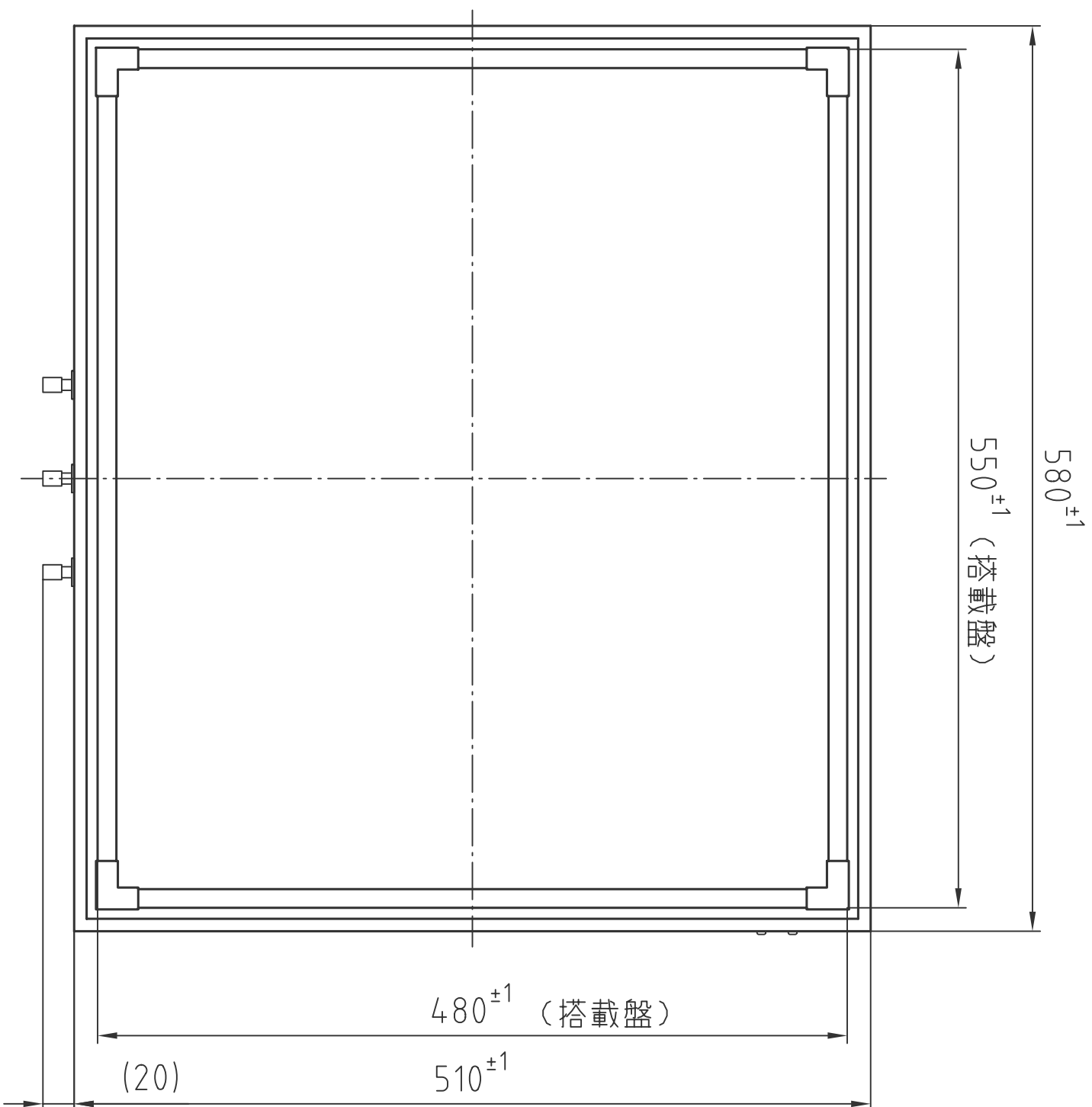
(平面図)
