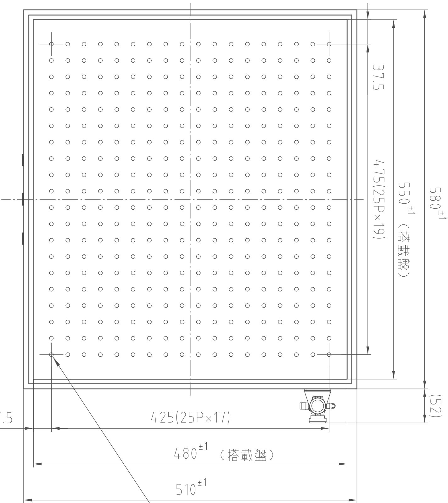
(平面図)
