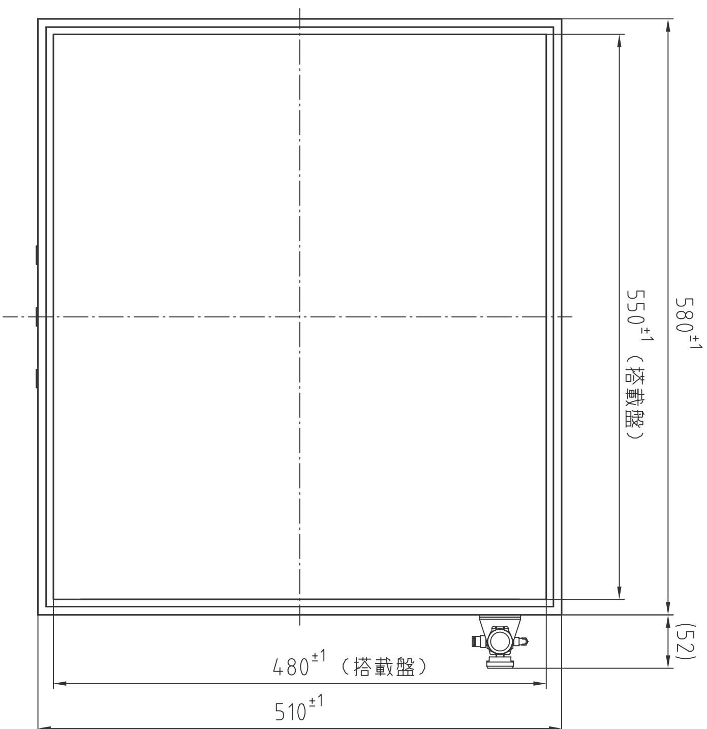
(平面図)
