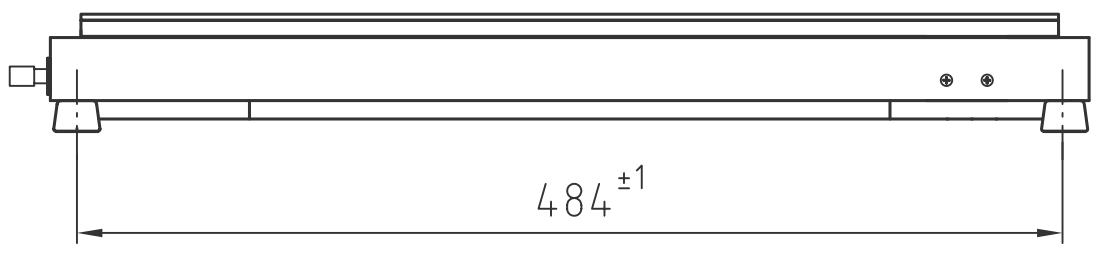
(右側面図)
