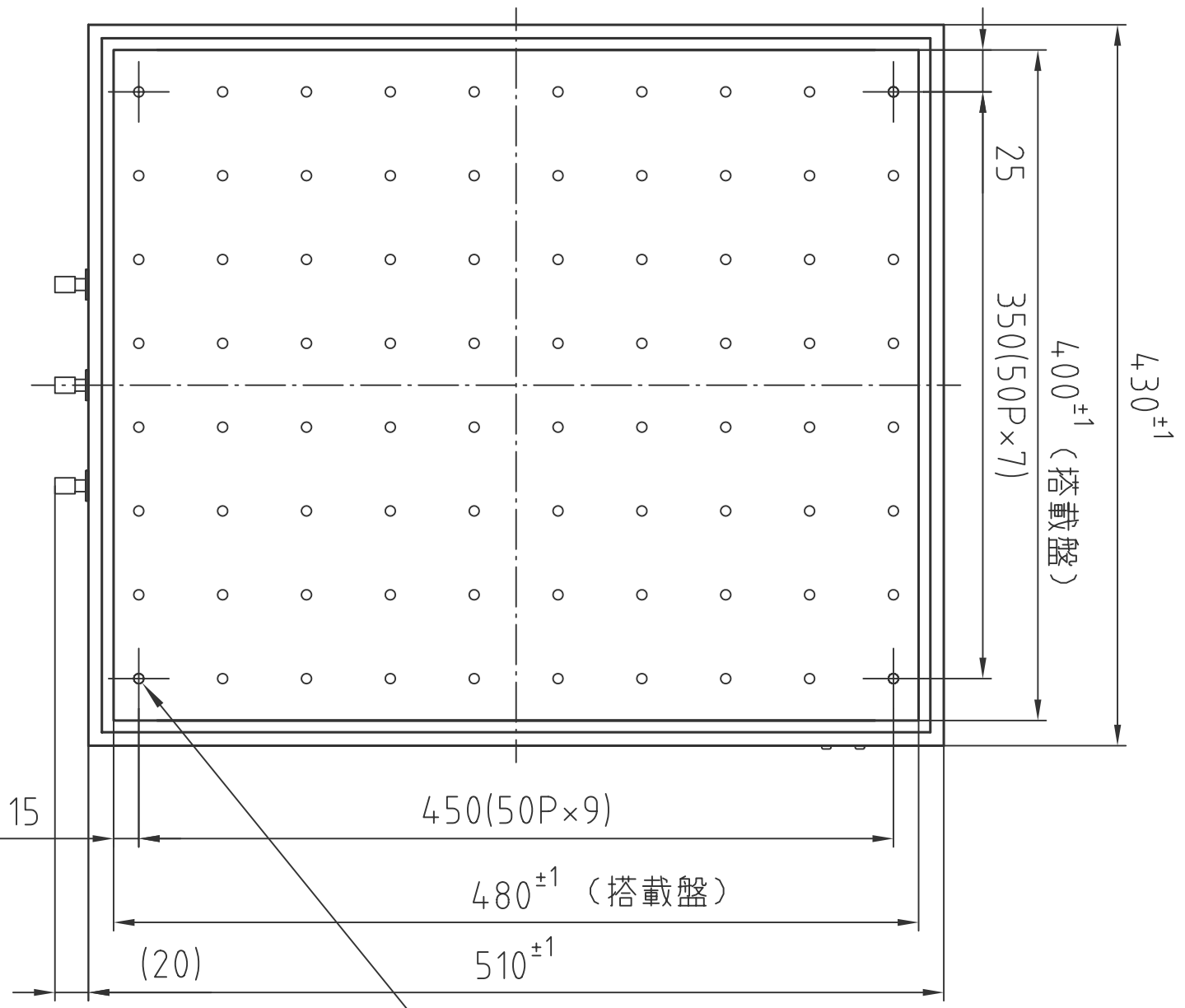
(平面図)
