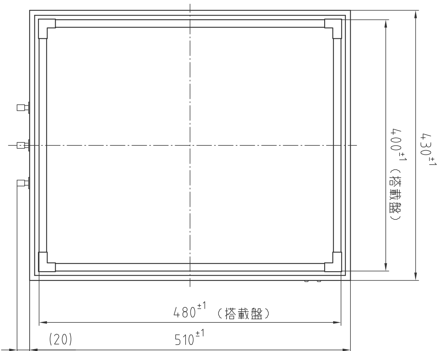
(平面図)
