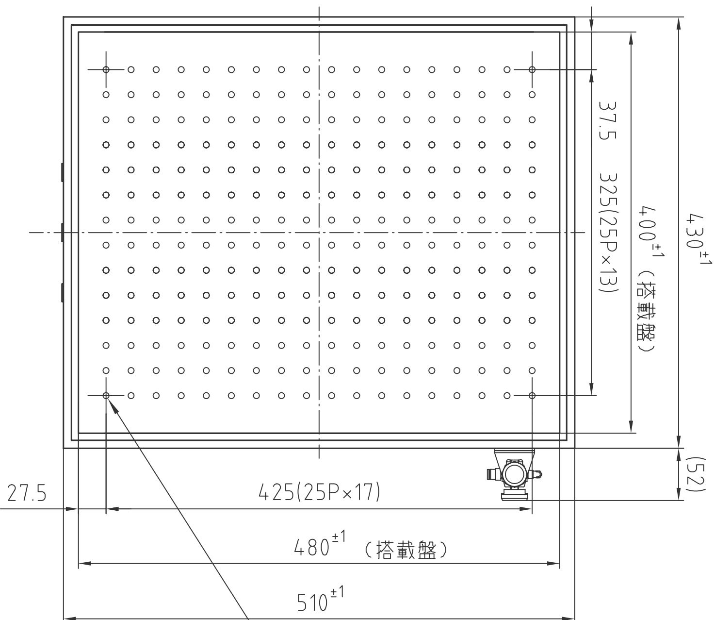
(平面図)
