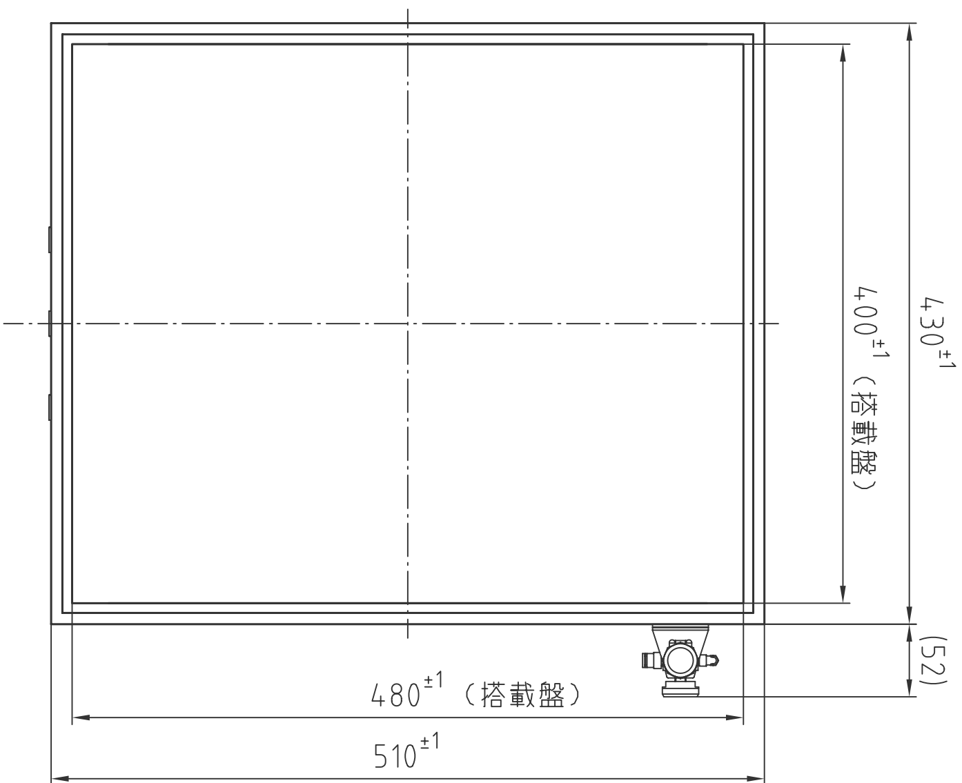
(平面図)
